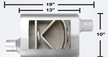
4"x10"x13" OFFSET/OFFSET
